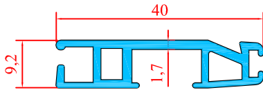
3289 0.380 Kg/m
