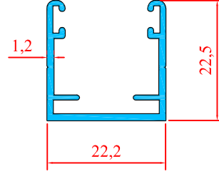
3286 0.252 Kg/m
