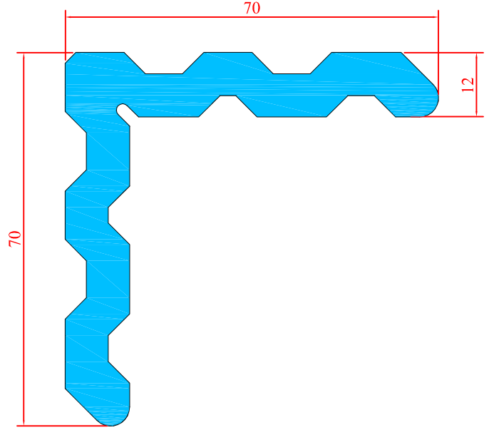
2126 3.310 Kg/m BAĞLANTI
